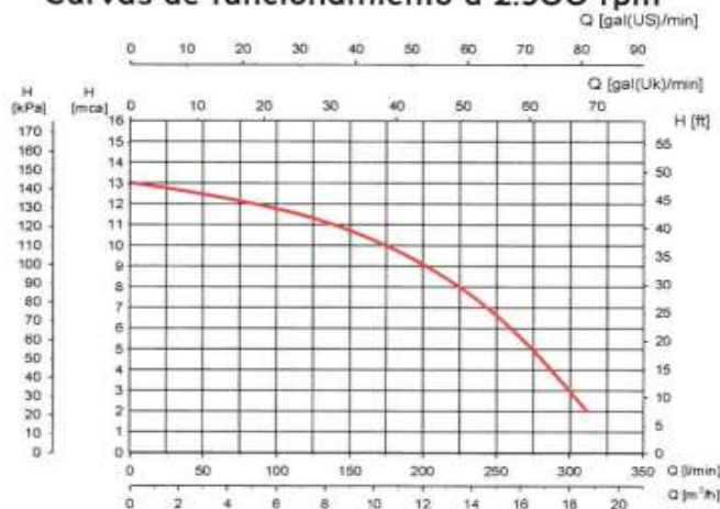
Curvas de funcionamiento a 2.900 rpm
